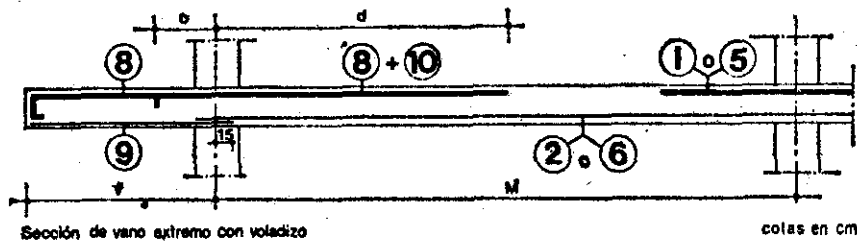
Sección de vano extremo con voladizo
