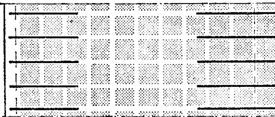
Planta armadura superior
