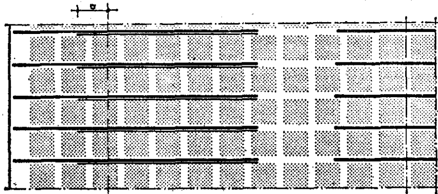
Planta armadura superior
