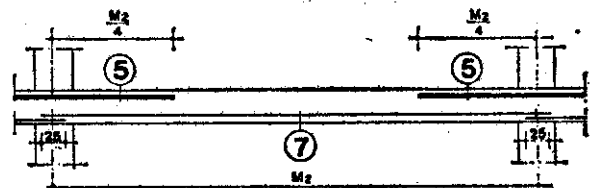
Sección vano interior
