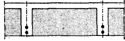
Al menos un redondo con \phi \geq 25
